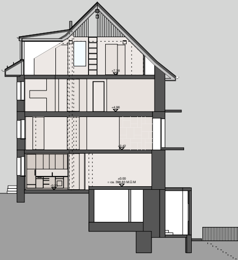
querschnitt 1-1
