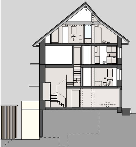
querschnitt 2-2
